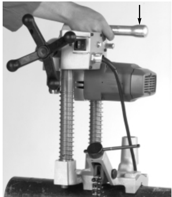
Figure 19 – Modèle HC-300 – Assemblage du moteur et de l'embase
