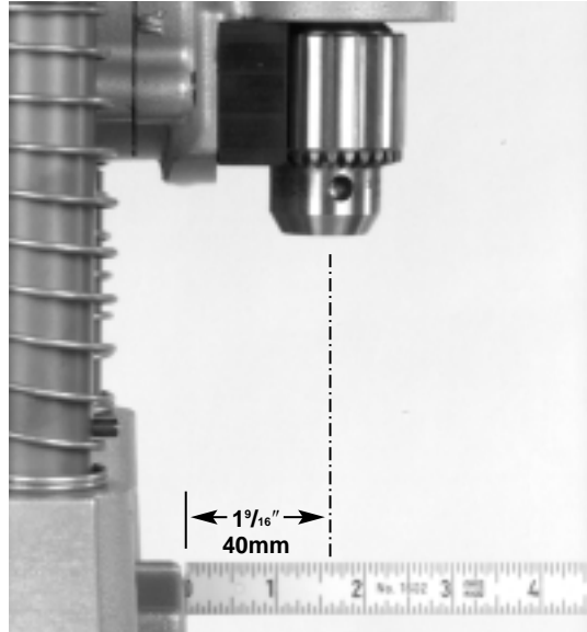
Figura 14 – Línea media del mandril de la HC-300
