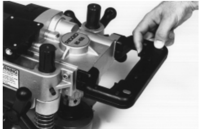
Figure 8 – Interrupteurs de verrouillage du modèle HC-450
