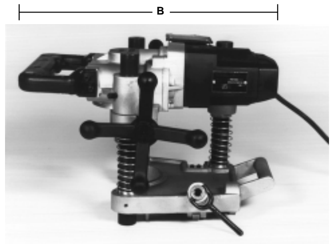
Figura 2 – Dimensión B
