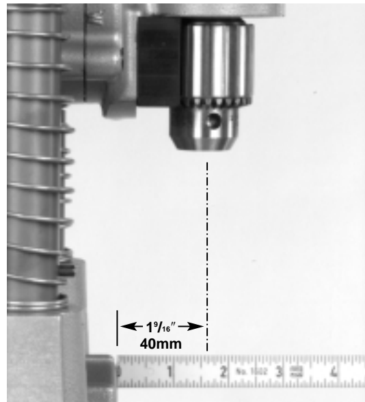
Figure 14 – Axe du mandrin de la HC-300
